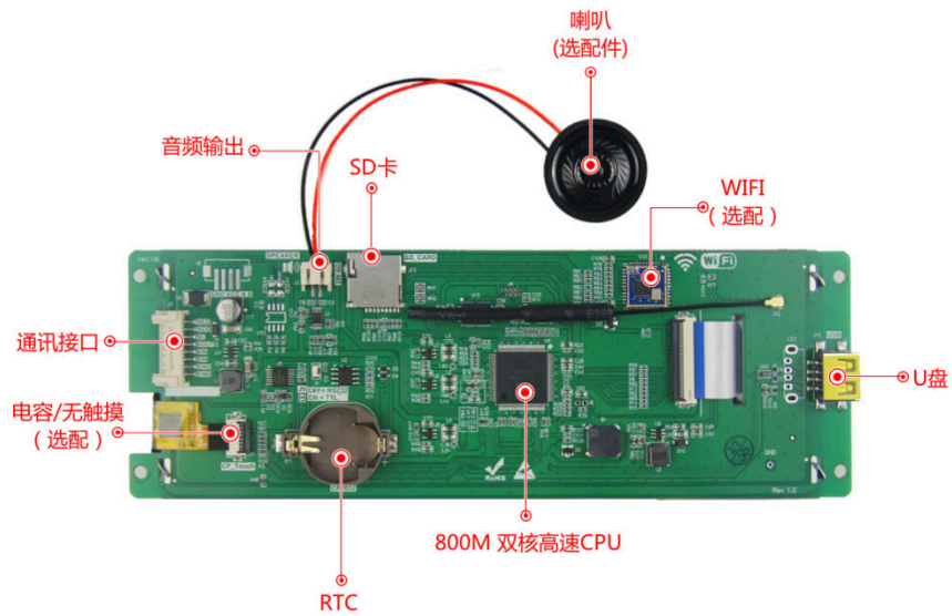
图 1-3 硬件配置图
